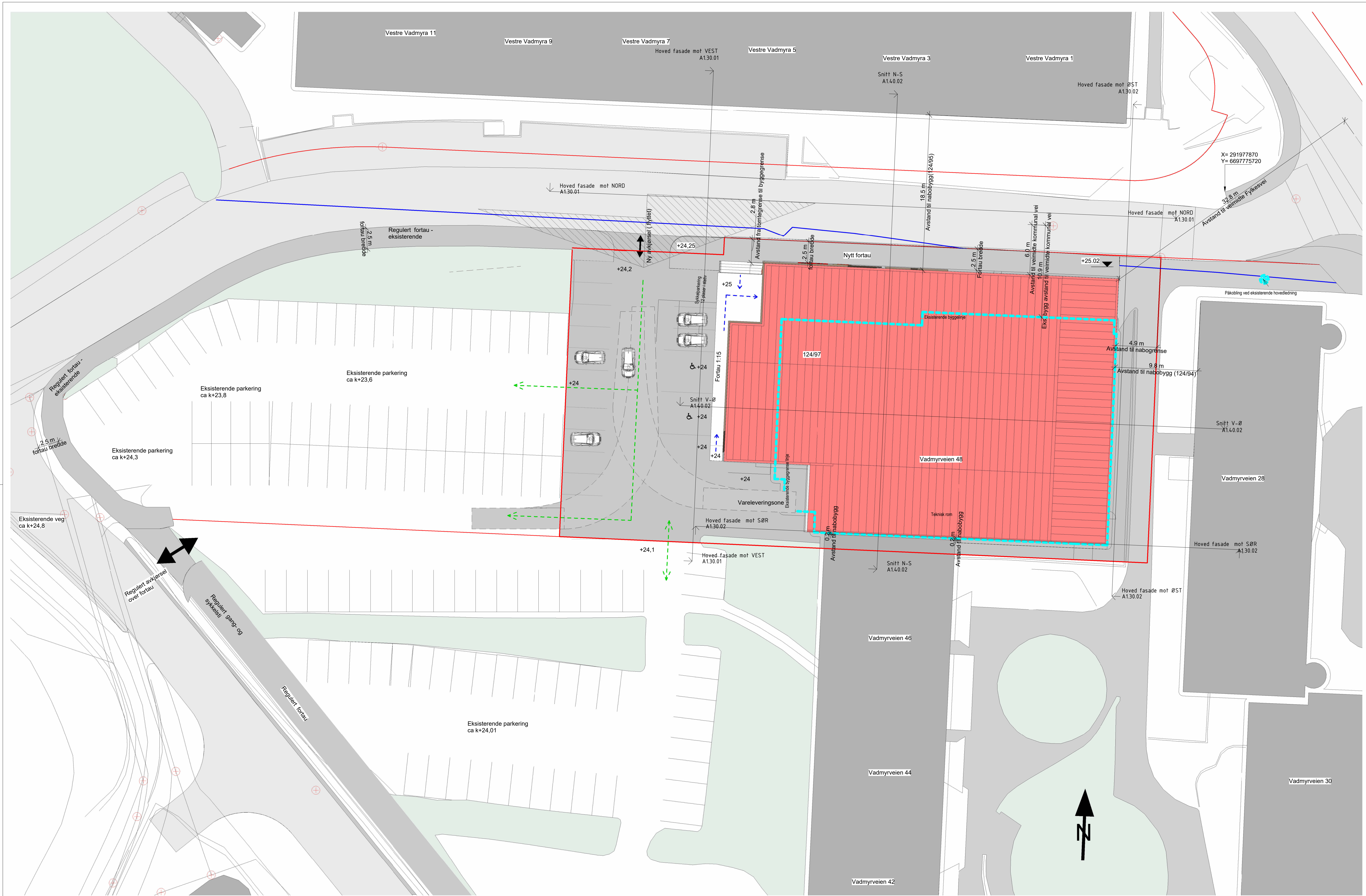
Ny Situasjonsplan 1 : 200
